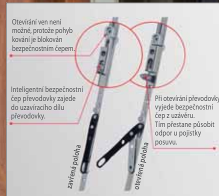
Štulpová převodovka
